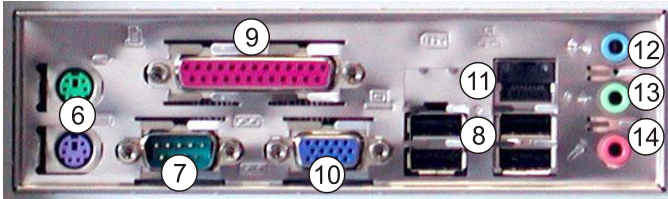
Detailansicht Anschlüsse, Beispielkonfiguration
