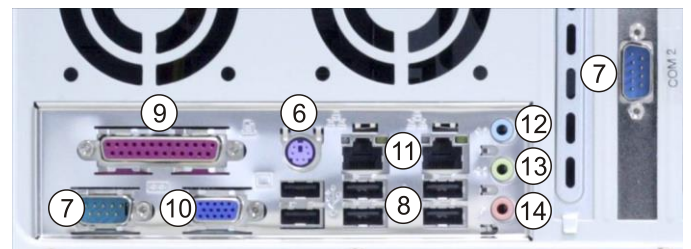
Rückansicht ATX-Mainboard-Version, Beispielkonfiguration
